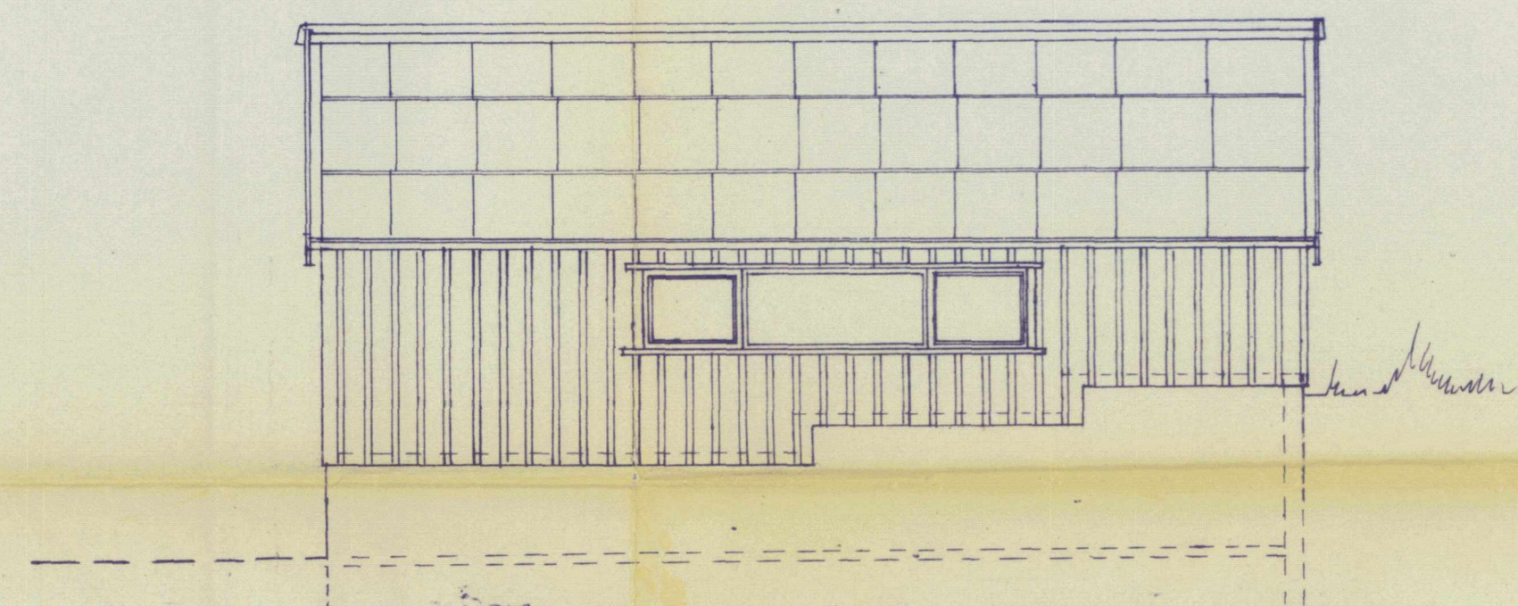
Fasade øst - M=1:50
