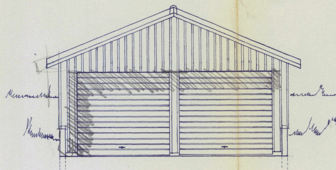
Fasade syd - M=1:50
