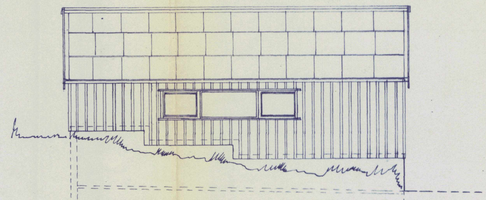
Fasade vest - M=1:50
