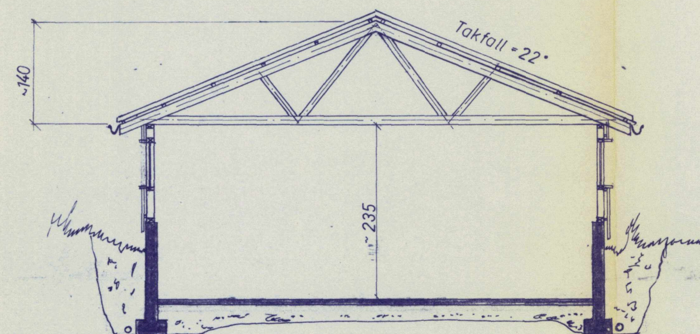
SNITT - M=1:50
