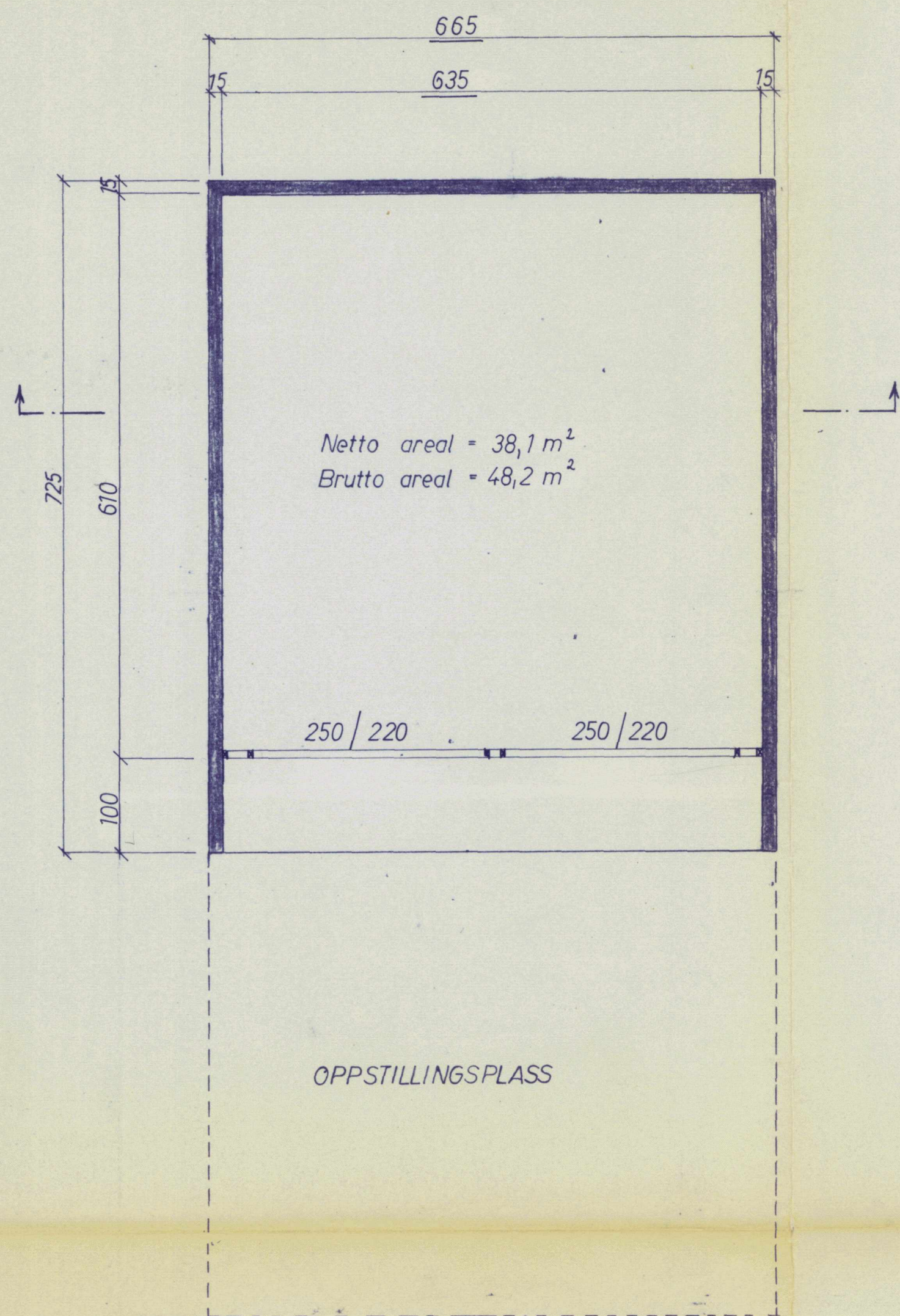
PLAN GARASJE - M=1:50
