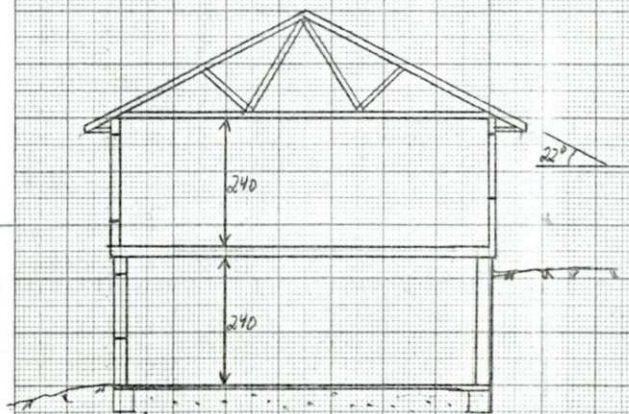
Snitt
