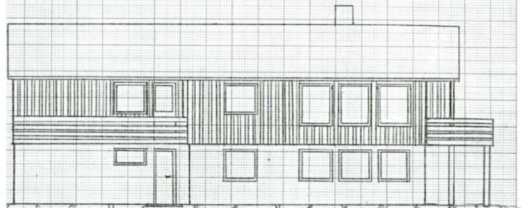
Fasade vest
