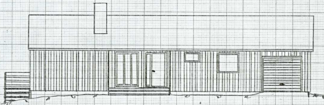
Fasade øst
