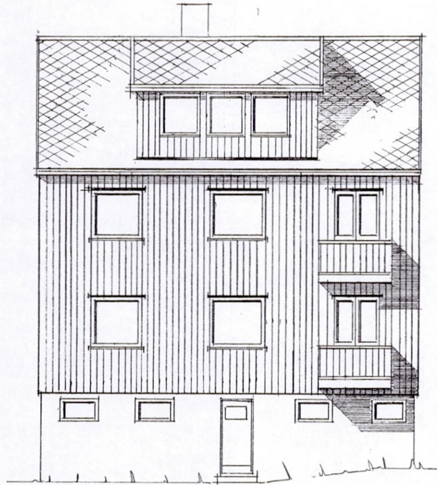
FASADE ØST
